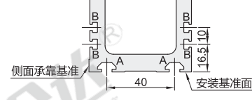
型材
