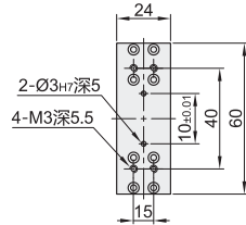
滑块(Z部放大图)
