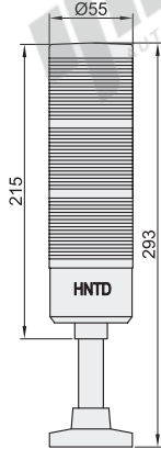
TD-55系列
