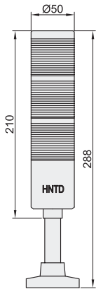
TD-50系列
