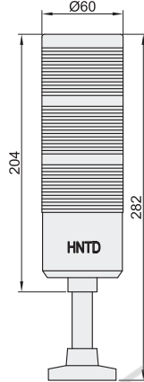
TD-60系列
