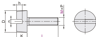
一字槽圆柱头螺钉 TAP31
