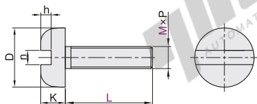
一字槽盘头螺钉 TAP25/26
