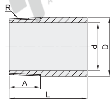
单头外螺纹 XLQ10
