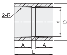
双头内螺纹 XLQ11
