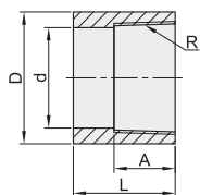
单头内螺纹 XLQ09
