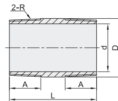
双头外螺纹 XLQ12
