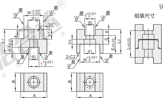
加长倒角凸台型 PDC21
