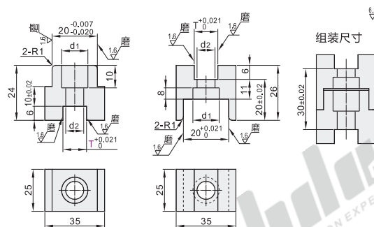
加长R角凸台型 PDC11
