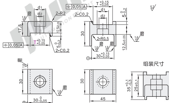
标准倒角凸台型 PDC16
