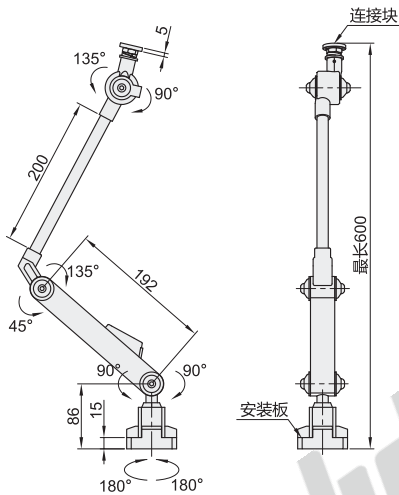
长度：M
