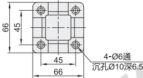
安装板尺寸
