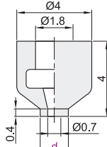
盘径Ø4
