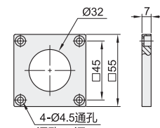
法兰尺寸
