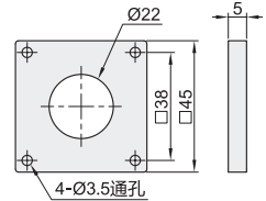
法兰尺寸
