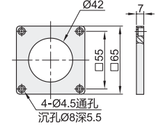
法兰尺寸
