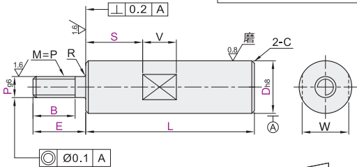
带扳手槽型 Y-FCH08
