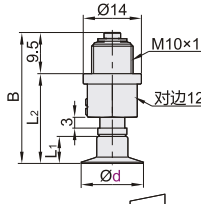
弹簧式直接安装型 J-WEU76/77
