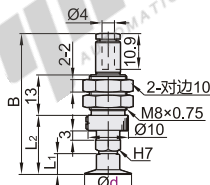
弹簧式顶部真空端口 J-WEU66/67
