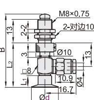
弹簧式侧面真空端口 J-WEU71/72
