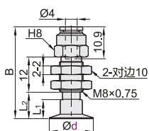
固定式顶部真空端口 J-WEU61/62
