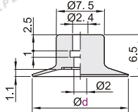
盘径Ø15
