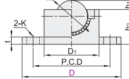
圆法兰式 QDA21
