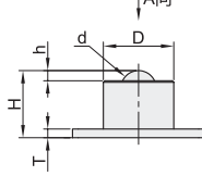
方法兰式 QDA20
