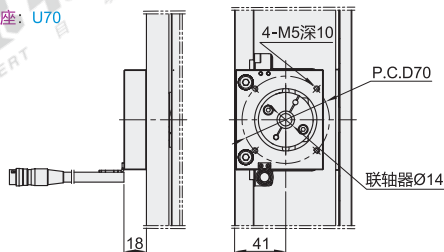
规格: 24024 电机安装座: U70
