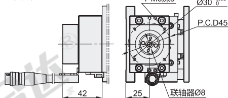
规格: 80100/12012 电机安装座: U45
