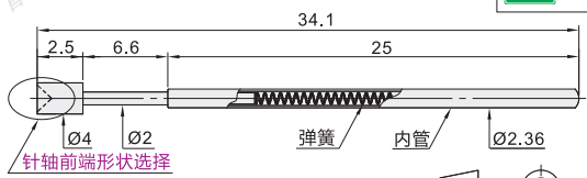
针轴前端形状
