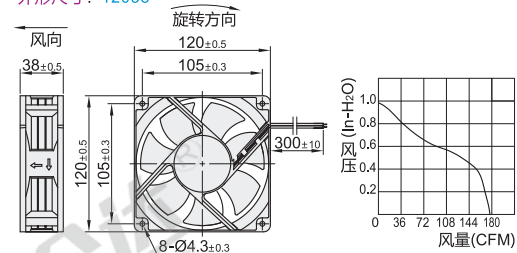
外形尺寸：12038
