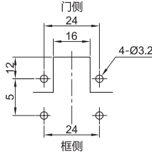
安装孔孔距
