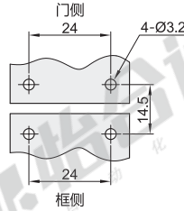
安装孔孔距
