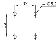
安装孔孔距
