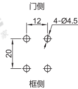
安装孔孔距
