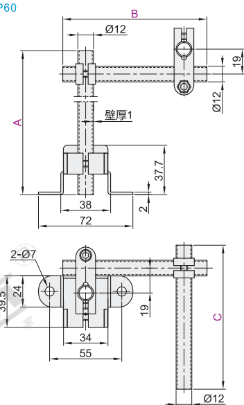
三管可调 ZLP60
