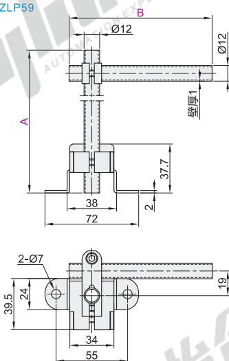
双管可调 ZLP59
