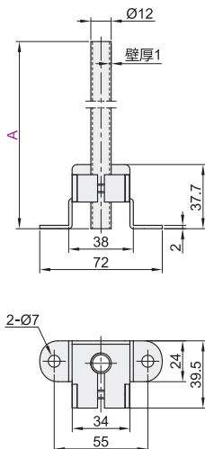
单管可调 ZLP58
