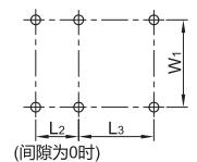
安装孔孔距
