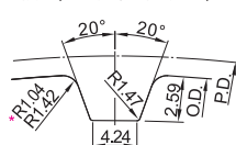
齿形 (ISO标准齿条尺寸)
