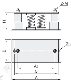
四弹簧型 NHF93
