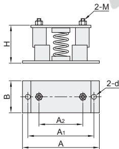
单弹簧型 NHF91
