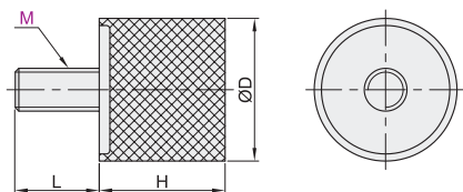
圆柱型 Y-RAE28
