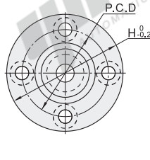
圆法兰 E-BFU61/62/63/66
