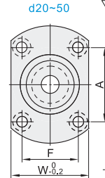
对边法兰 E-BFU81/82/86
