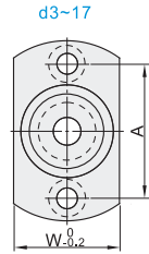
对边法兰 E-BFU81/82/86
