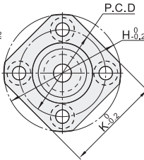
方法兰 E-BFU71
