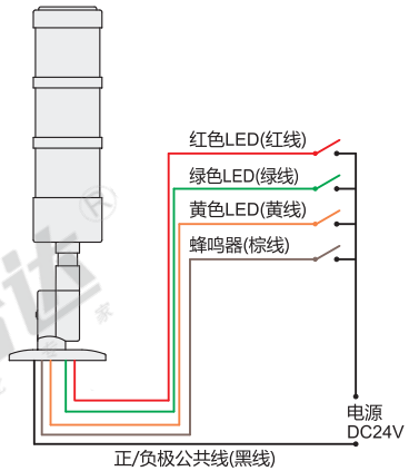
接线图
