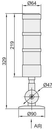
底盘安装尺寸(共用)
