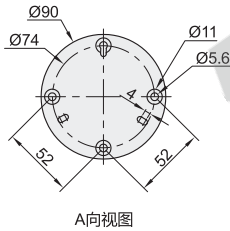
底盘安装尺寸(共用)
