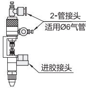
装配示意图
