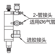
装配示意图
