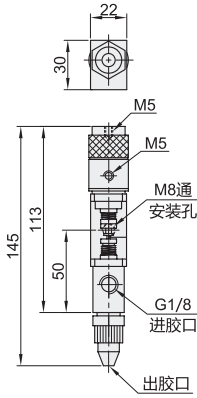
装配示意图
