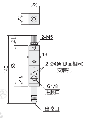
装配示意图
