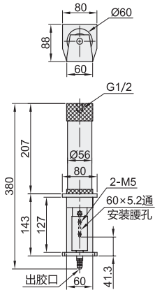
装配示意图
