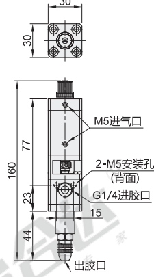
装配示意图
