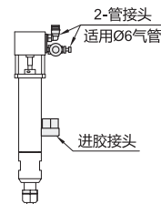
装配示意图
