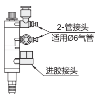
装配示意图
