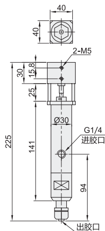
装配示意图
