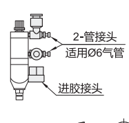
装配示意图
