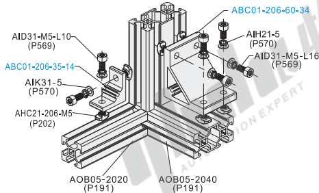
分解图
