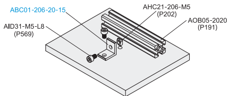
分解图
