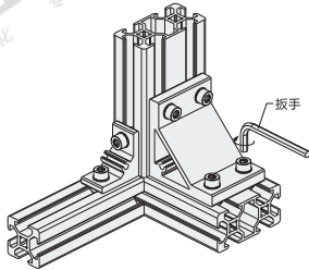
组装图
