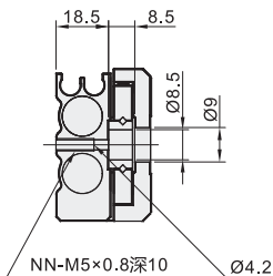
截面A-A
