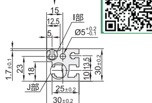
型材截面放大图 传送面侧
