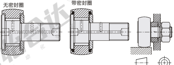
全滚针球面型 E-BPC27
