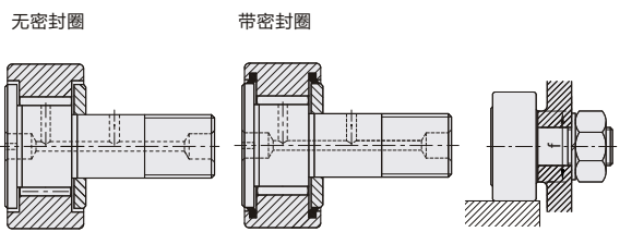
全滚针圆柱型 E-BPC07
