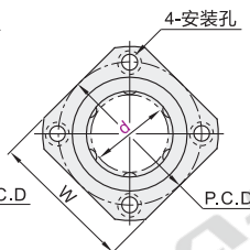
方法兰型 J-LMP12
