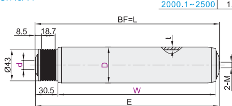
内螺纹型 QCH43/44
