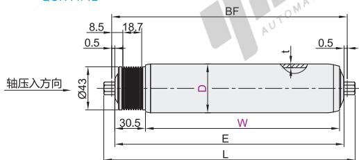
弹簧压入式 QCH41/42
