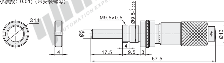
EPD25 (行程: 0~13)(最小读数: 0.01) (带安装螺母) 球头测量面
