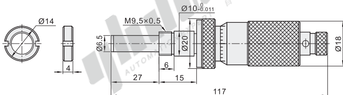
EPD43(行程: 0~25)(最小读数: 0.01) (带安装螺母)
