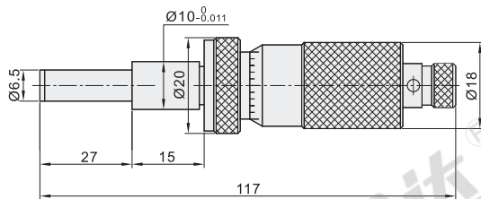
EPD43(行程: 0~25)(最小读数: 0.01) (带安装螺母)
