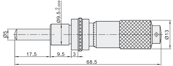
EPD22 (行程: 0~13)(最小读数: 0.01)
