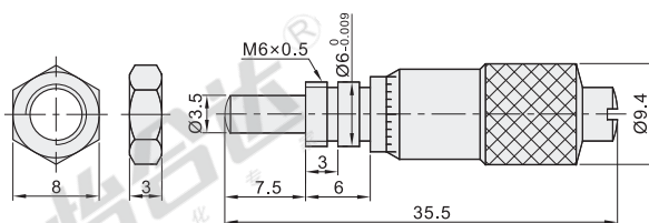
EPD02 (行程: 0~6.5)(最小读数: 0.01)
