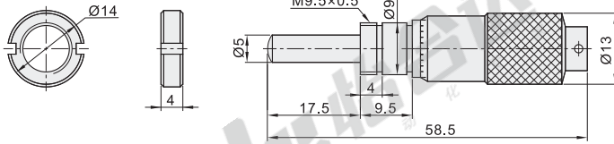
EPD24 (行程: 0~13)(最小读数: 0.01) (带安装螺母)
