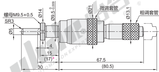
EPD27(行程: 粗调0~13; 微调0~0.2)(最小读数: 粗调0.01; 微调0.0005) (带安装螺母)
