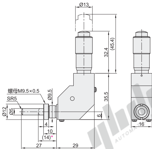
EPD25 (行程: 0~13)(最小读数: 0.01) (带安装螺母) 球头测量面
