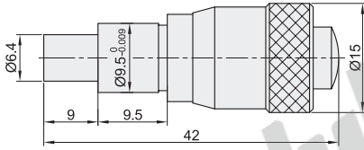
EPD21 (行程: 0~13)(最小读数: 0.01)
