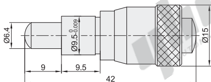
EPD05 (行程: 0~6.5)(最小读数: 0.01)
