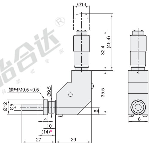
EPD26 (行程: 0~13)(最小读数: 0.01) 平头测量面
