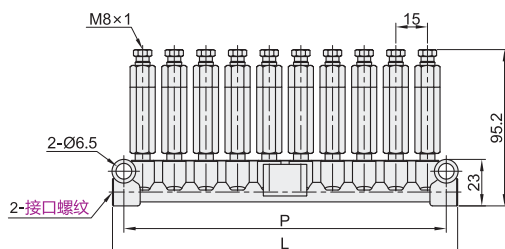
卸压型 WTB02
