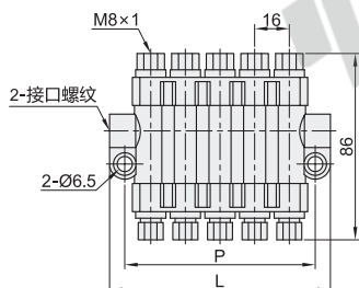
标准型 WTB01
