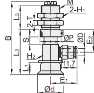
盘径 \varnothing 15 \sim 50
