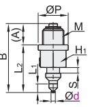
盘径 \varnothing 2 \sim 4
