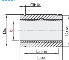
封闭型 Y-GSB31
