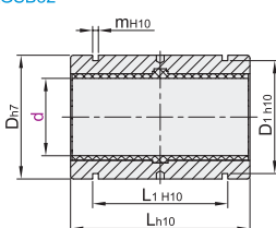
开口型 Y-GSB32
