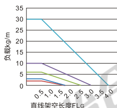
直线架空长度与负载关系图FLG
