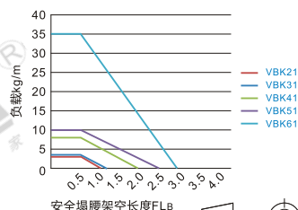
安全塌腰架空长度与负载关系图FLB
