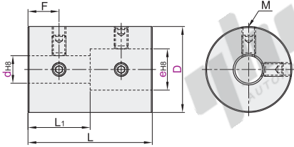
螺钉固定型 DCP11
