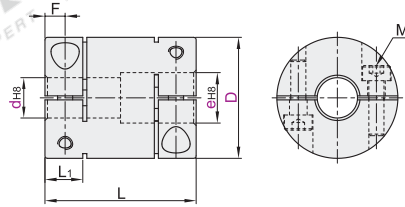
螺钉夹紧型 DCP13
