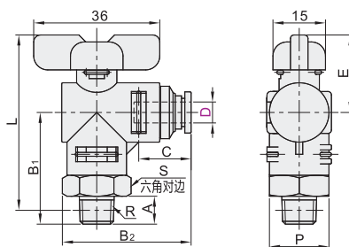
弯管型 J-XYK61
