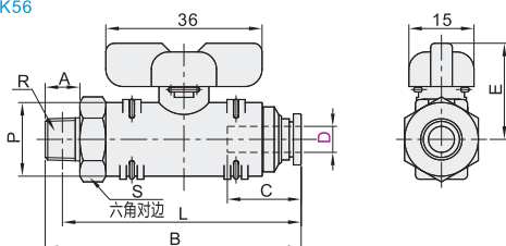
直管型 J-XYK56
