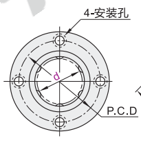
圆法兰型
