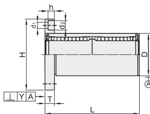
双衬型
