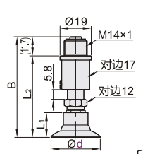
弹簧式直接安装型 J-WET76/77
