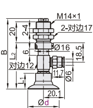
弹簧式侧面真空端口 J-WET71/72
