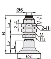
固定式顶部真空端口 J-WET61/62
