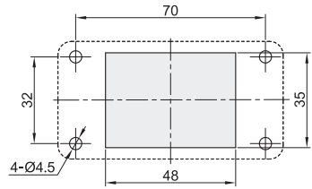
■ 面板开孔图
