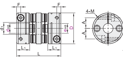
双膜片 DBM22
