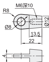
前端形状接头 (活塞杆端与气缸筒端接头)
