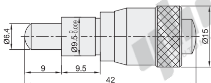
EPD05 (行程: 0~6.5)(最小读数: 0.01)
