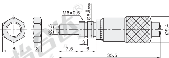
EPD02 (行程: 0~6.5)(最小读数: 0.01)
