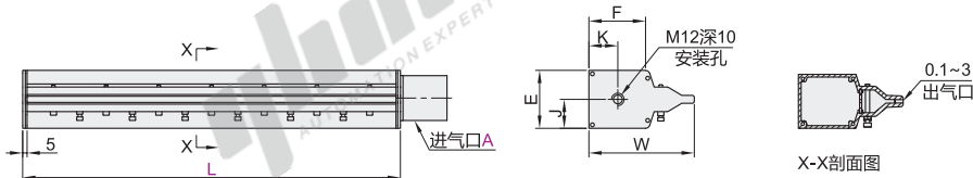
X-X剖面图
