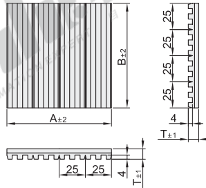
突起详图
