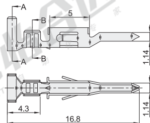
5558系列-端头 39-00-0040
