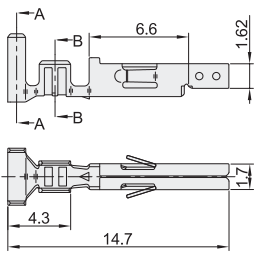
5556系列-端头 39-00-0038
