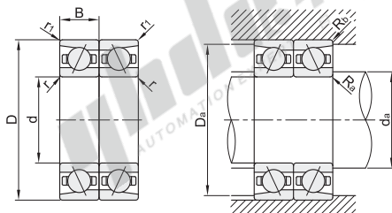
安装图
