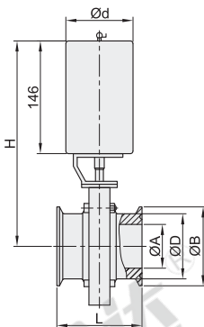
立式 BLA93
