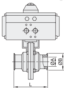
卧式 BLA90/91
