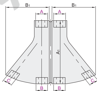
展开视图
