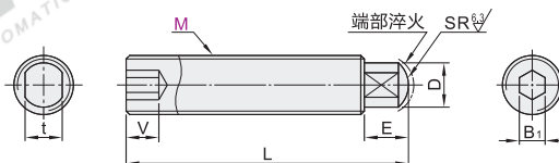
内六角孔带扳手槽型 PAS31/32/36/37
