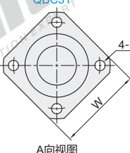
方法兰式 QDC31
